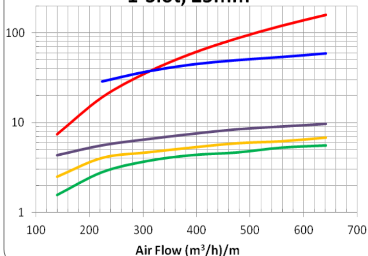
1-Slot, 25mm
